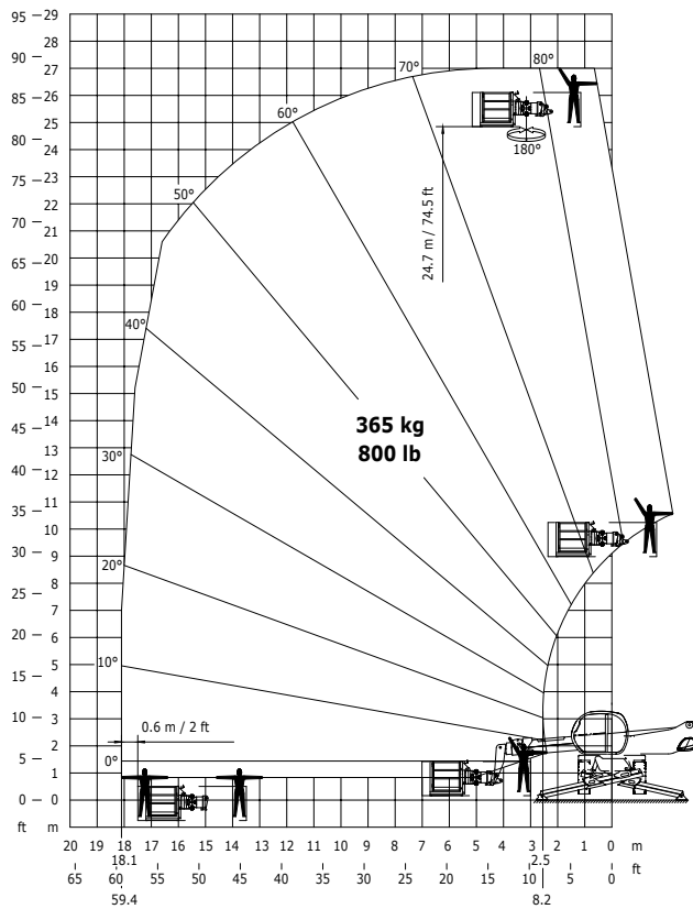
Věž vytočená, stabilizační patky spuštěny s navijákem 5000kg
