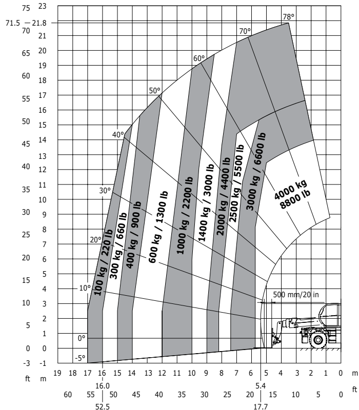
Věž v přímé pozici na kolech s vidlicemi
