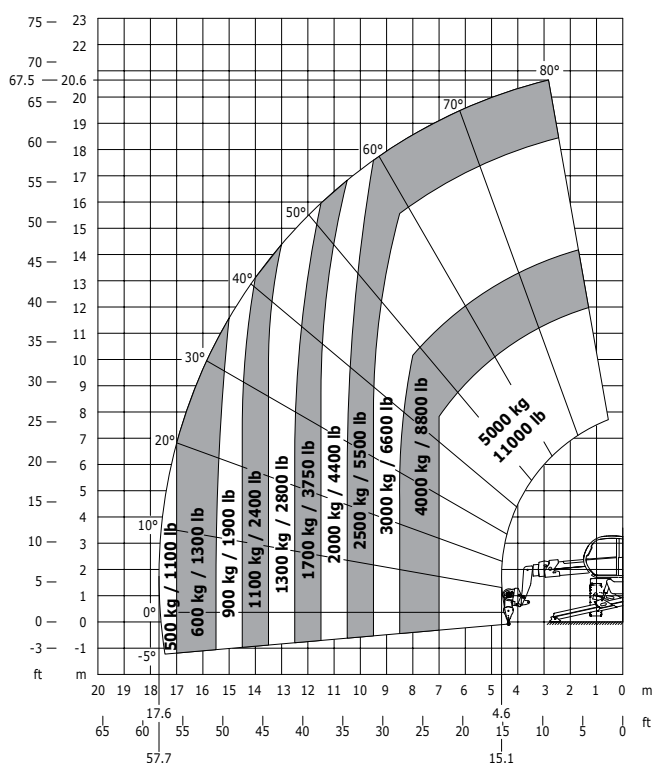
Věž vytočená, stabilizační patky spuštěny s navijákem 5000kg
