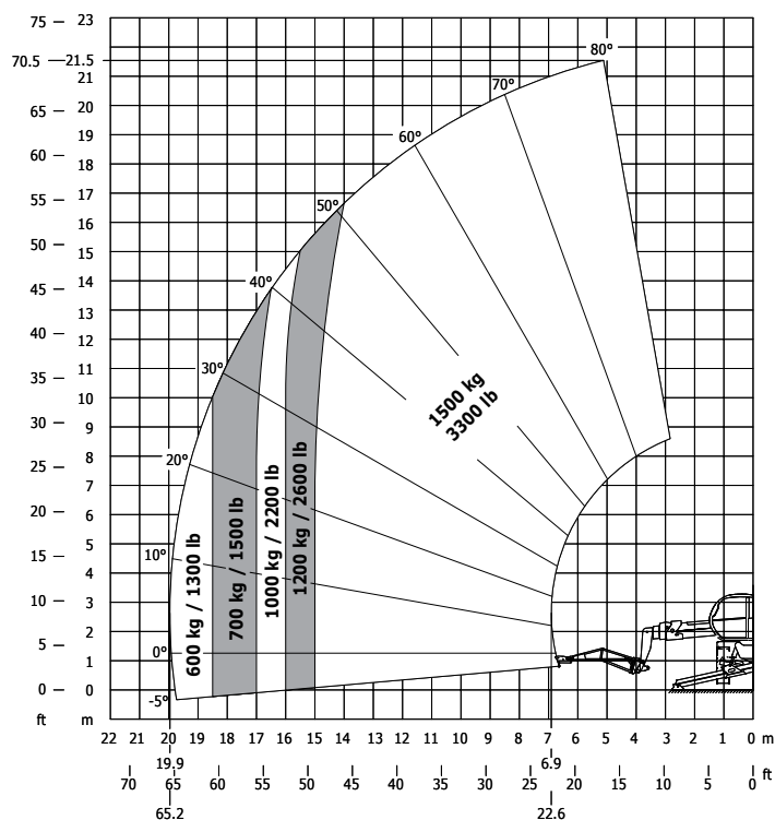
Věž vytočená, stabilizační patky spuštěny s jeřábovým hákem 1500mm
