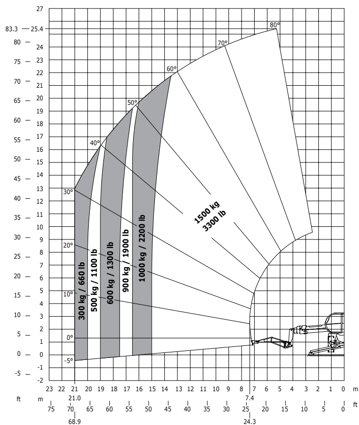
Věž vytočená, stabilizační patky spuštěny s jeřábovým hákem 1500mm
