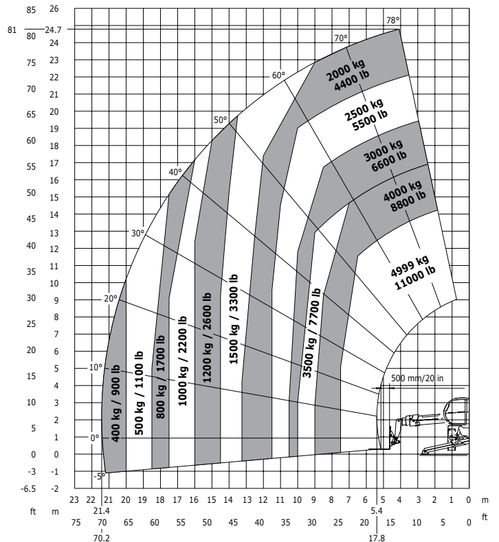
Věž vytočená, stabilizační patky spuštěny s vidlicemi
