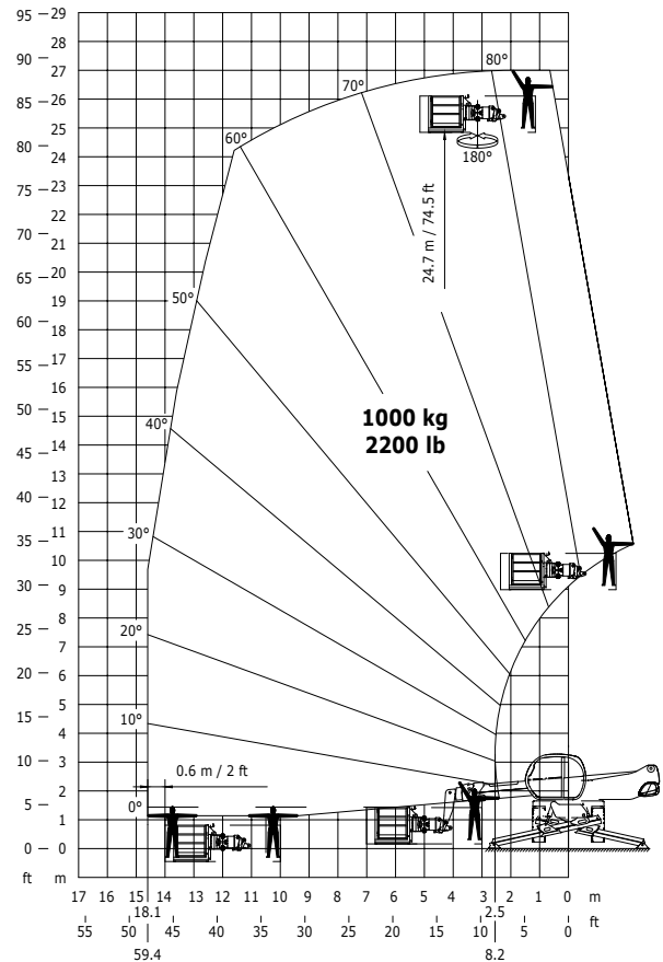
Věž vytočená, stabilizační patky spuštěny s pracovní plošinou 1000kg
